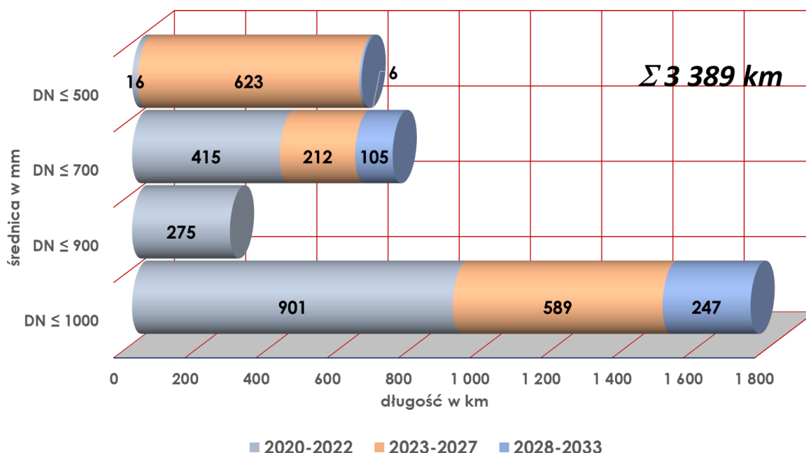
Wykres 4 Efekty rzeczowe realizacji Planu Rozwoju na lata 2020-2033 – przyrost długości sieci przesyłowej
